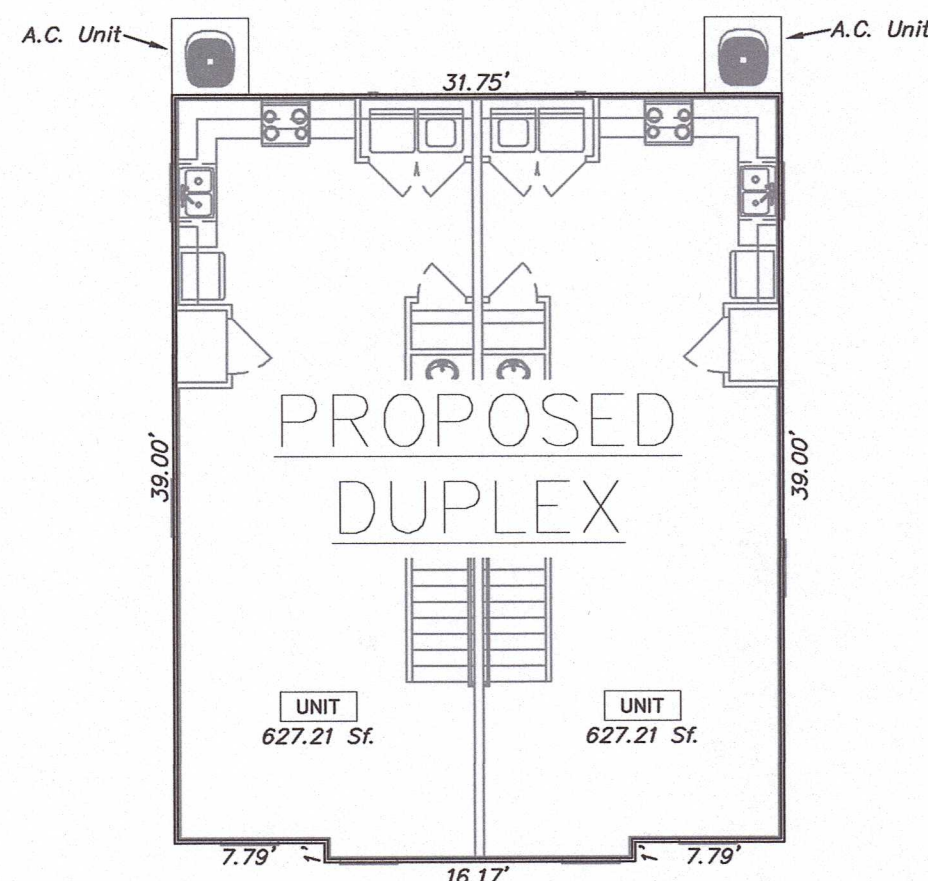
TYPICAL PROPOSED DUPLEX (N.T.S.)
